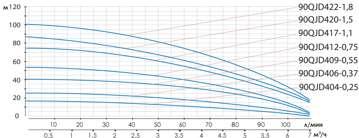
График 4. Расходно-напорные характеристики насосов 90QJD404-0,25 - 90QJD422-1,8 (высо-та-объемная подача).
