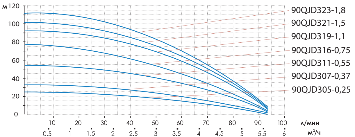
График 3. Расходно-напорные характеристики насосов 90QJD305-0,25 - 90QJD323-1,8 (высота-объемная подача).
