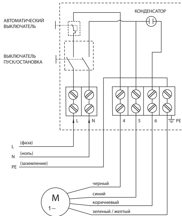
Рис. 4. Электрическая схема.
