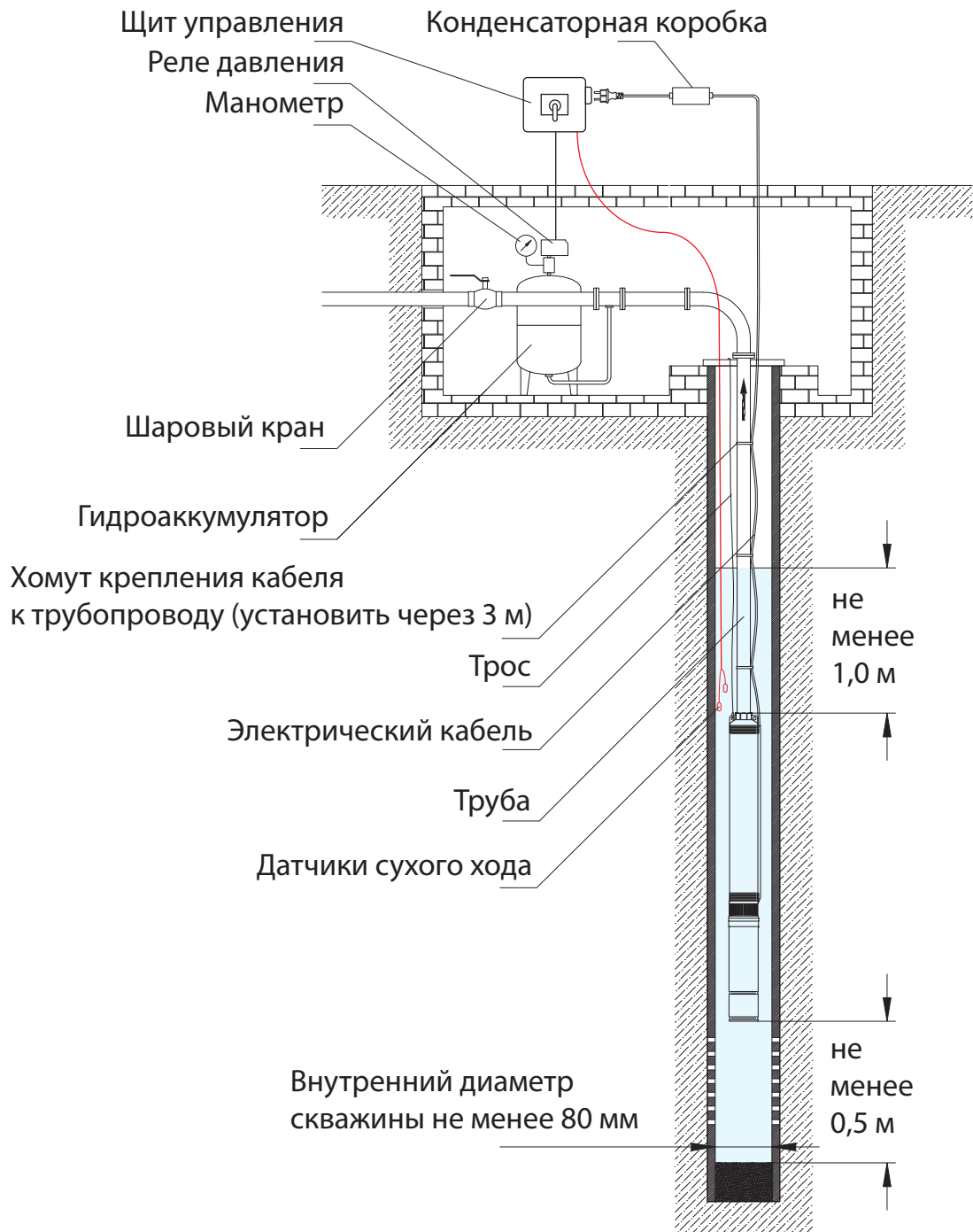
Рис. 1. Схема установки электронасоса в скважину.
