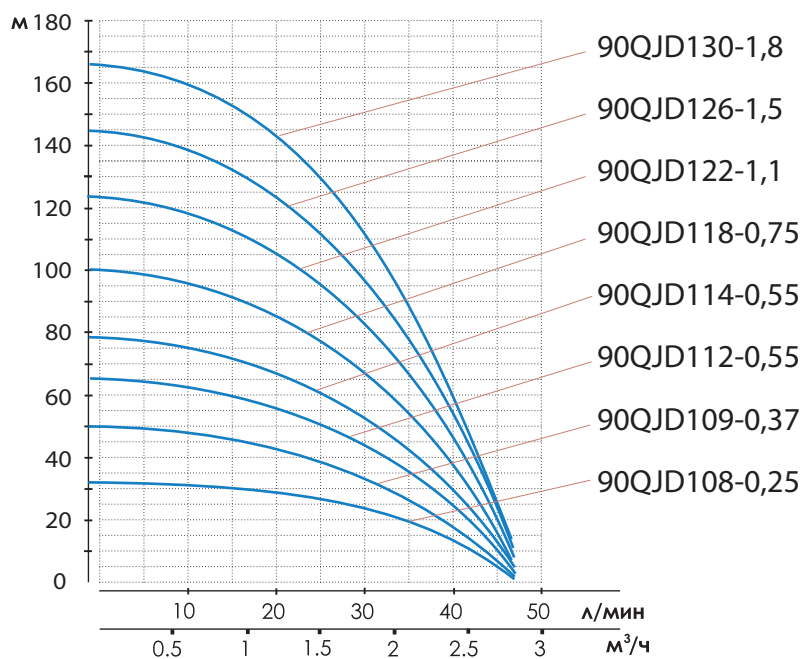
График 1. Расходно-напорные характеристики насосов 90QJD106-0,25 - 90QJD130-1,8 (высота-объемная подача)
