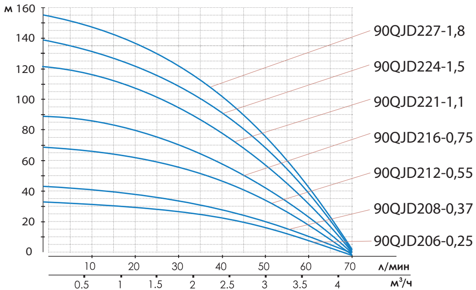
График 2. Расходно-напорные характеристики насосов 90QJD206-0,25 - 90QJD227-1,8 (высота-объемная подача).
